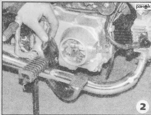
Рис. 40. Регулировка сцепления
