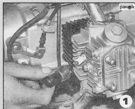
Рис. 25. Замена свечи зажигания
