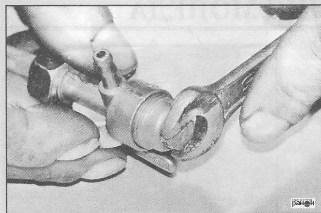
Рис. 4. Разборка топливного крана во время технического обслуживания
