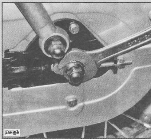
Рис. 30. Натяжение приводной цепи
