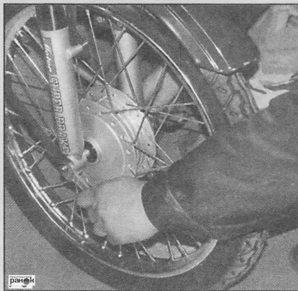
Рис. 36. Снятие колеса
