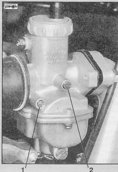
Рис. 27. Расположение регулировочных винтов карбюратора: 1 - винт регулировки состава смеси (винт качества); 2 - винт регулировки частоты вращения коленчатого вала на холостом ходу (винт количества)
