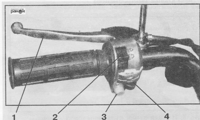
Рис. 7. Левая ручка руля: 1 - рычаг выключения сцепления; 2 - переключатель дальнего света фары; 3 - кнопка звукового сигнала; 4 - переключатель указателя поворотов
