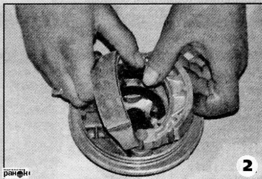
Рис. 38. Замена тормозных колодок
