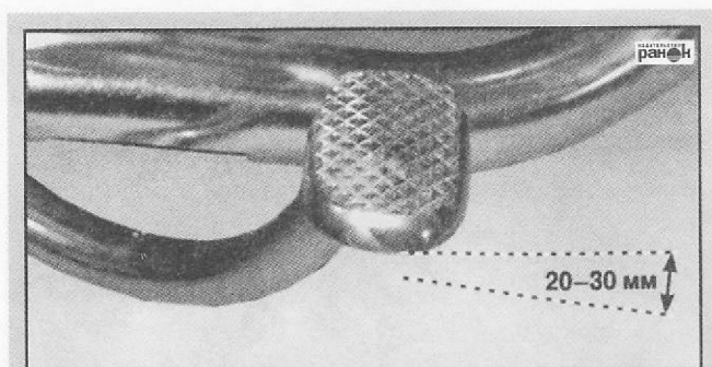
Рис. 33. Свободный ход педали заднего тормоза
