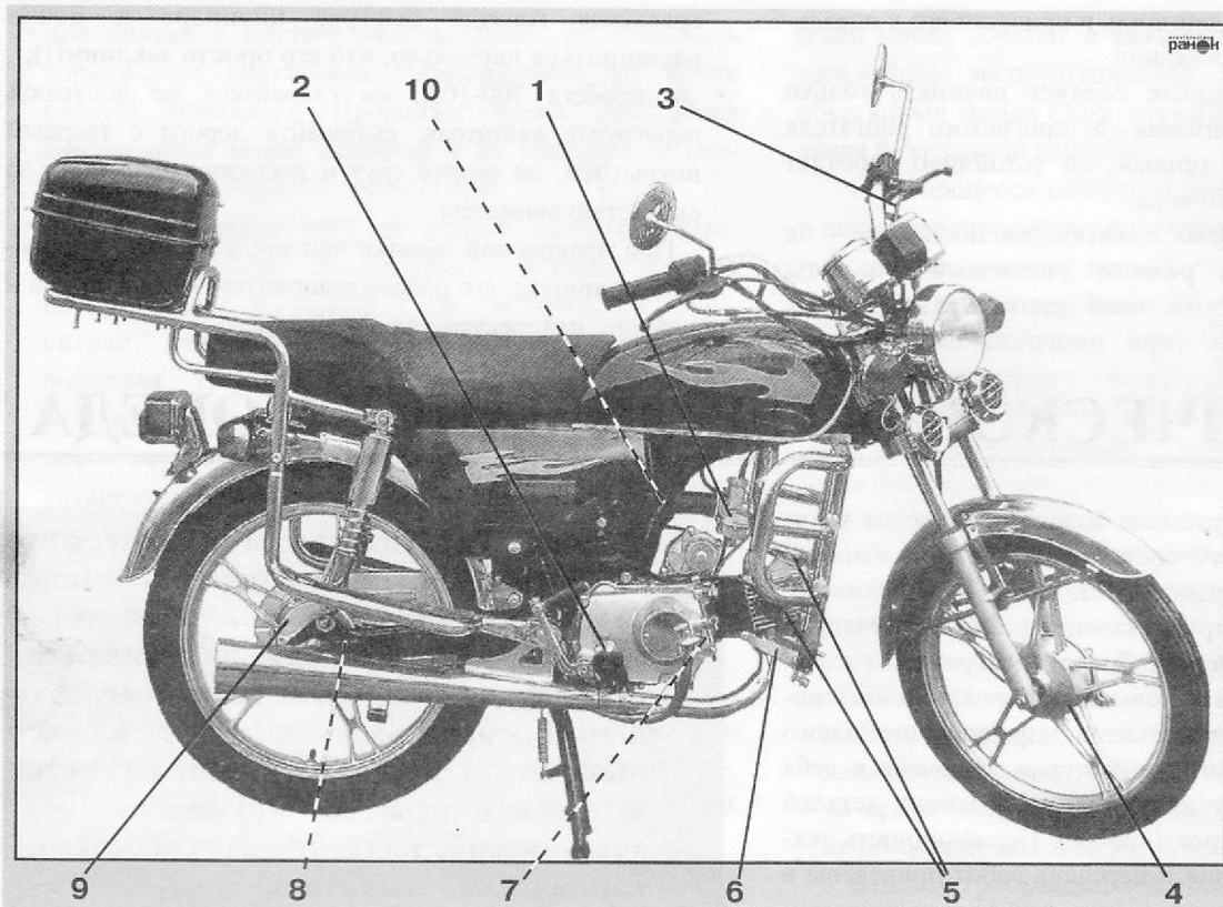
Рис. 12. Расположение основных элементов обслуживания mopeda:
