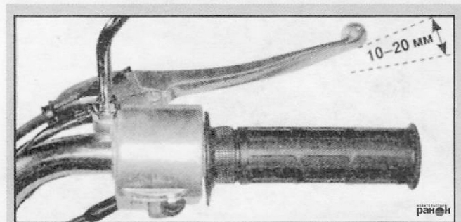
Рис. 31. Свободный ход рычага переднего тормоза
